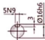
入力軸
