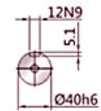
入力軸
