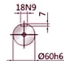
入力軸
