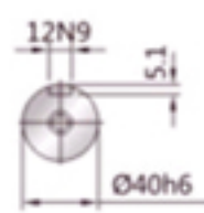
出力軸
