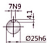
入力軸
