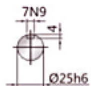
入力軸
